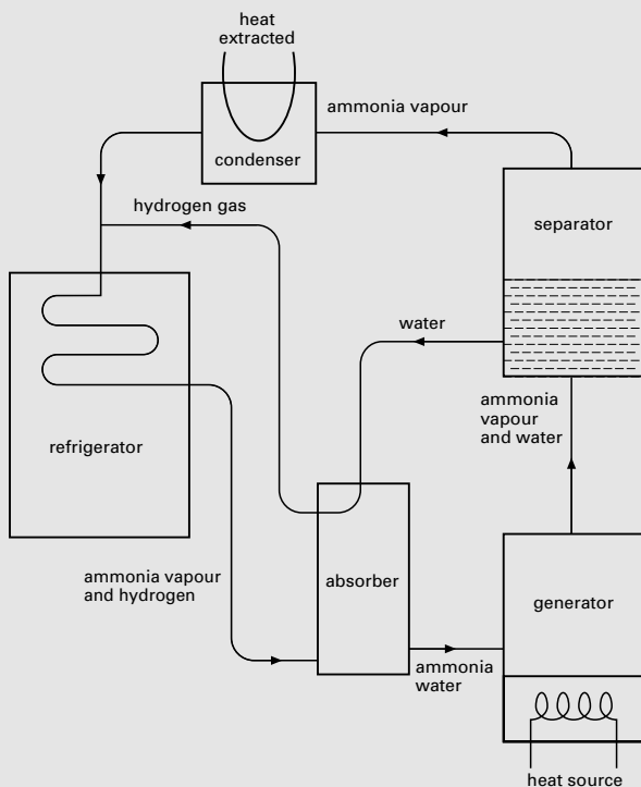
Vapour-absorption cycle
