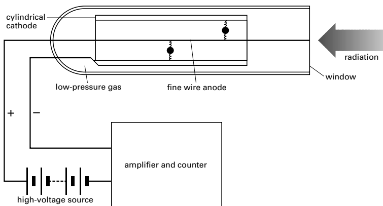
Geiger counter
