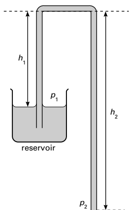
Siphon
