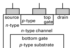
JFET
