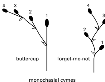
monochasial cymes
