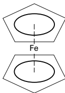
Ferrocene
