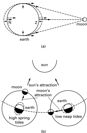
Tides
